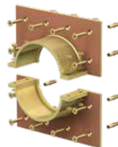
Variante : Tube fourreau Curaflex® 8000/T sablé
